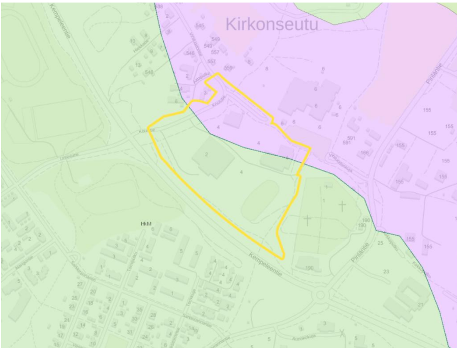
Kuva 5 Maaperäkartta. Vaalean vihreällä hiekkaa olevat alueet, vaalean violetilla hienoa hietaa olevat alueet.
